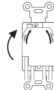
3. Turn module to lock Tourner le module pour le verrouiller Gire el módulo para bloquear
