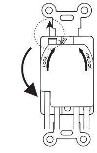
4. Push latch up and turn to release Pousser le loquet vers le haut et tourner pour libérer Empuje el seguro y gire para liberar
