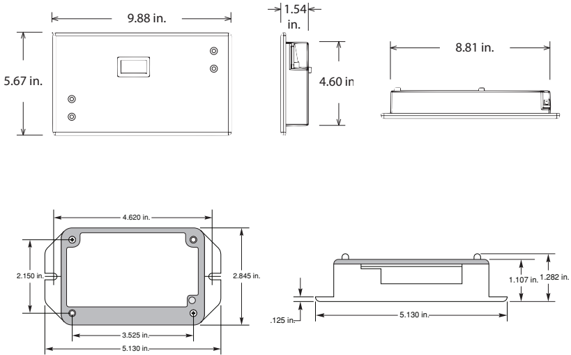
Figure 1 - Mini Meter flush mount enclosure dimensions
