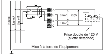
Dia. 2 Bipolaire à trois fils 120/240 V c.a.
