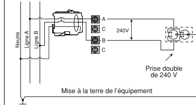
Dia. 1 Bipolaire à deux fils 120/240 V c.a.
