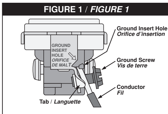
WIRING DIAGRAM 1 SCHÉMA DE CÂBLAGE 1
