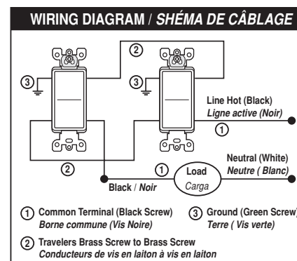
WIRING DIAGRAM 2 SCHÉMA DE CÂBLAGE 2
