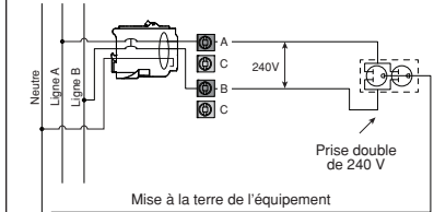
Dia. 1 Bipolaire à deux fils 120/240 V c.a.
